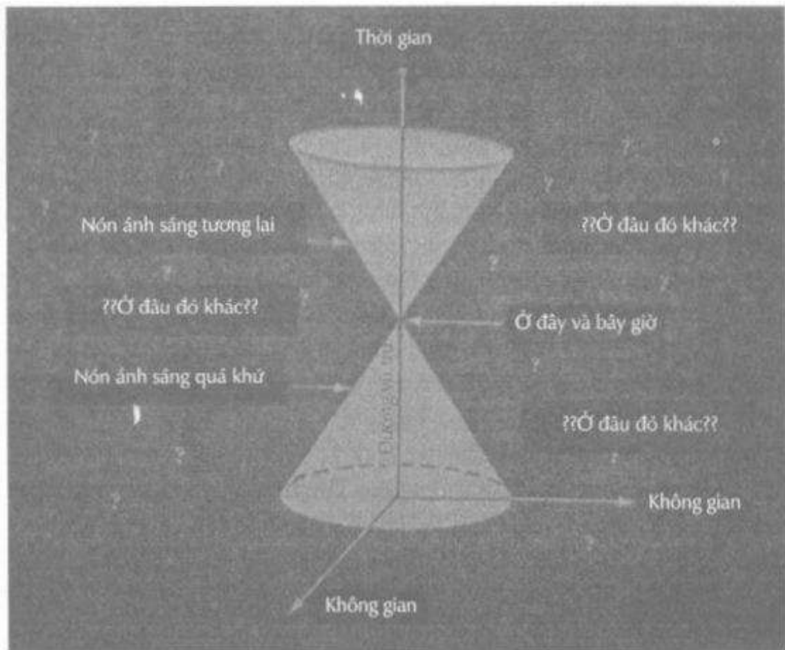
Hình 17.3. Hình nón ánh sáng của không-thời gian.
